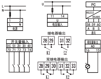
接线示意图
