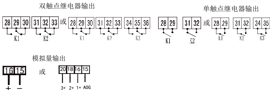
接线示意图
